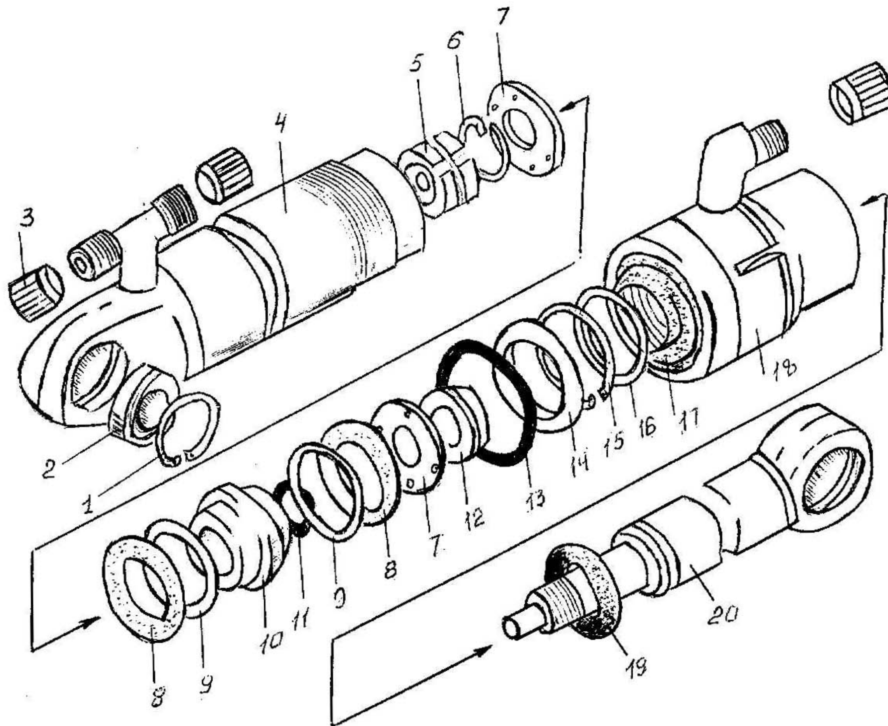
Рис. 9. Гидроцилиндр рукояти правый
