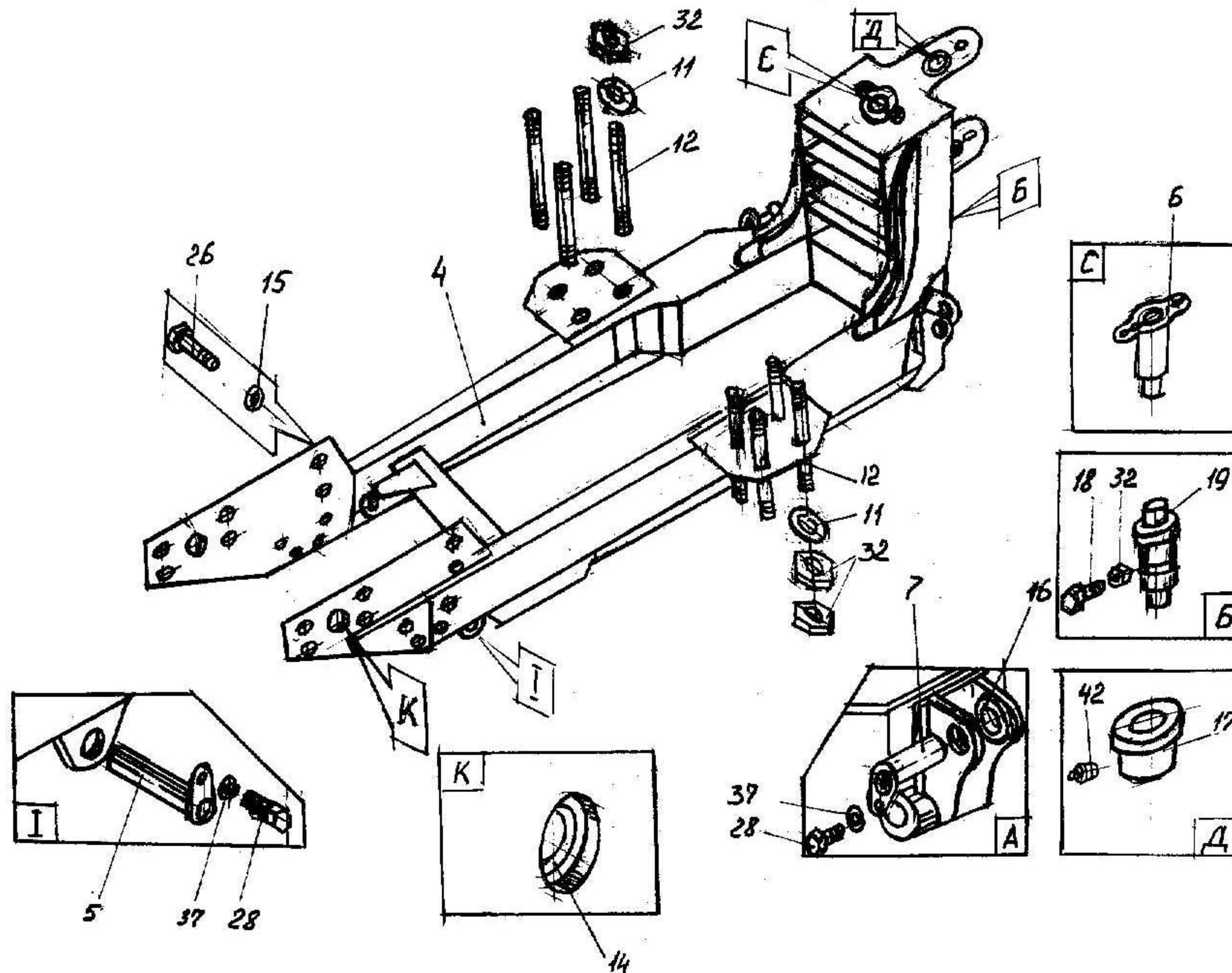
Рис. 3 Рама
