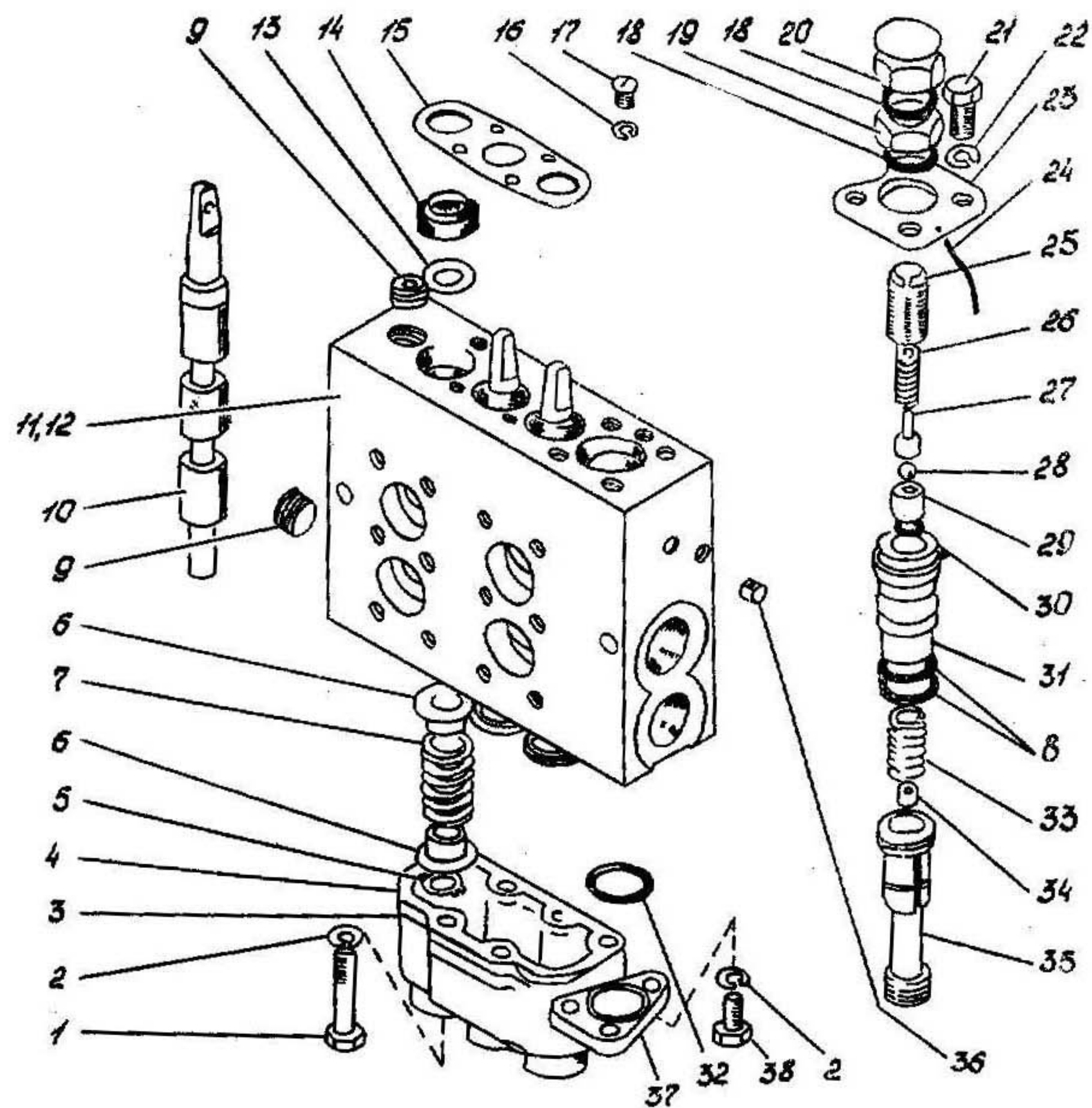
Рис. 25. Гидрораспределитель
