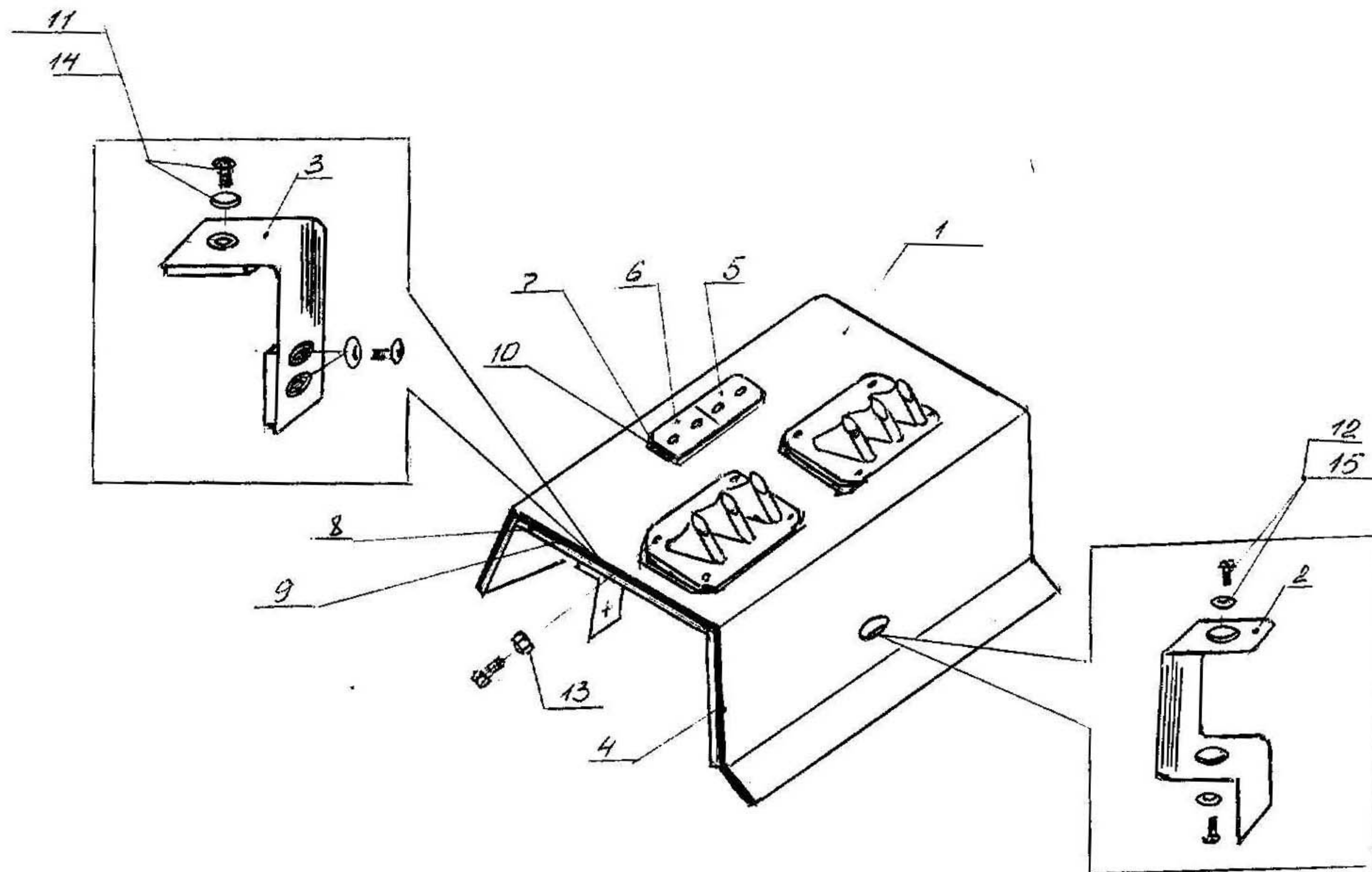
Рис. 21. Щиток управления
