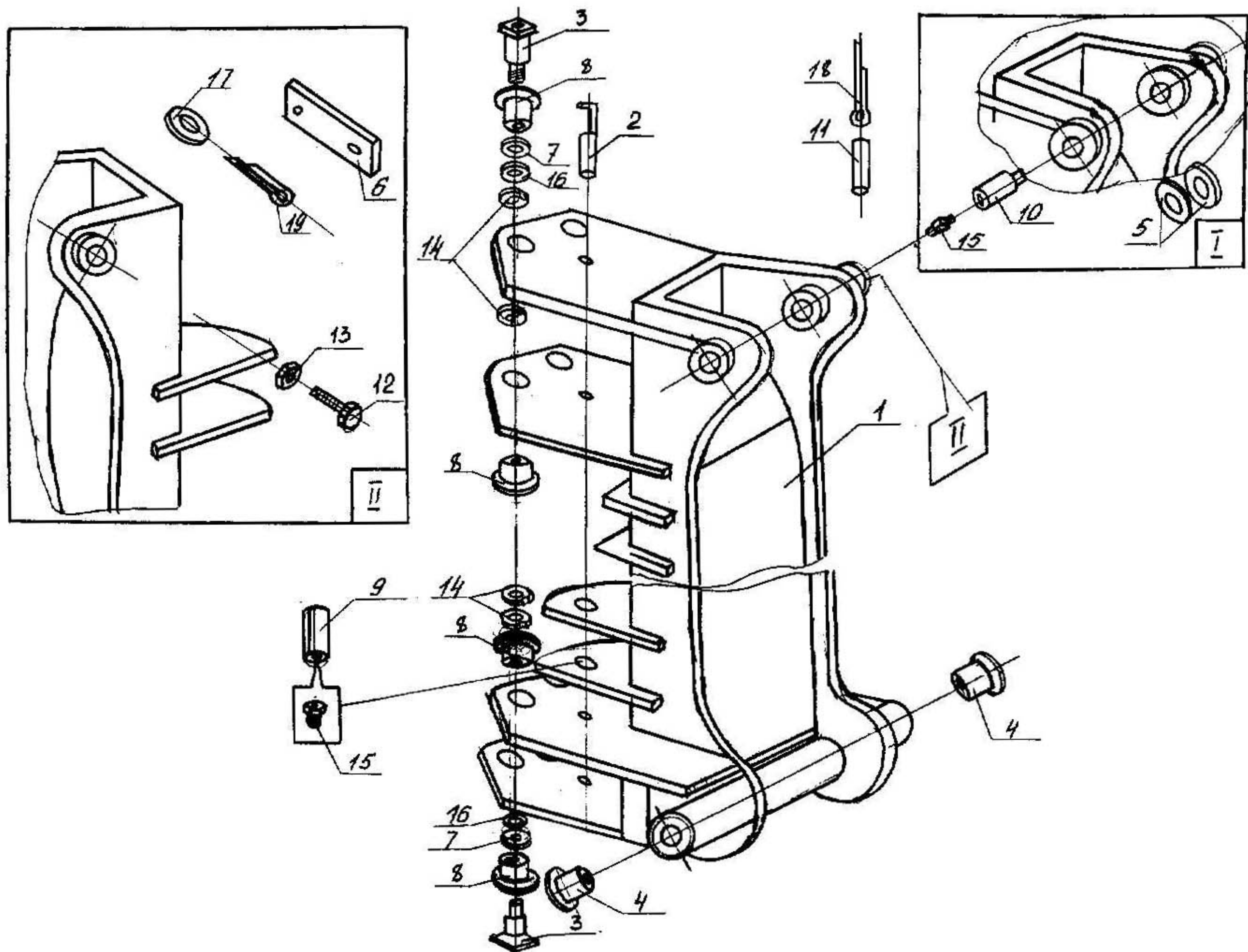
Рис. 6 Колонка
