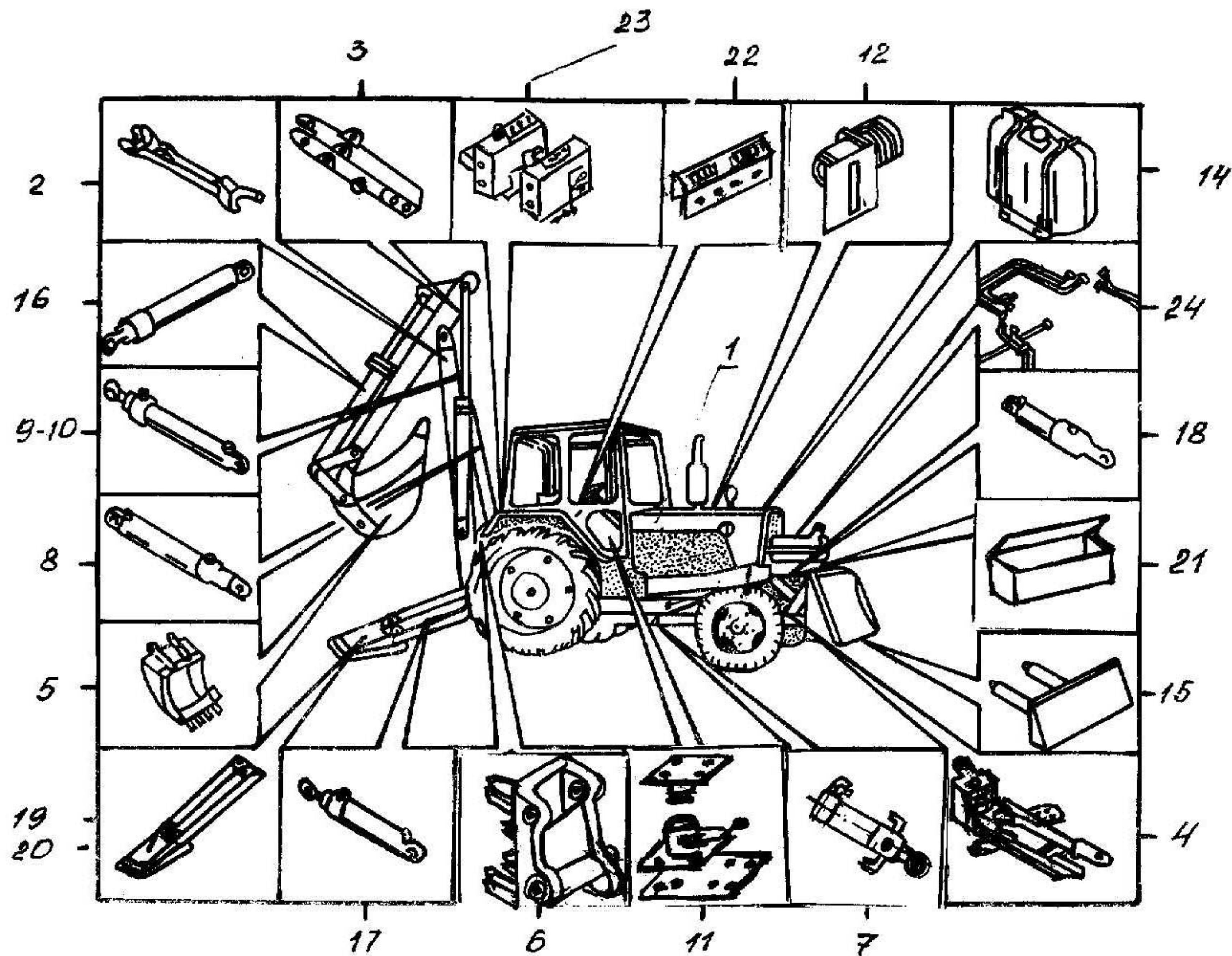
Экскаватор ЭО-2621В3 (на тракторе МТЗ)
