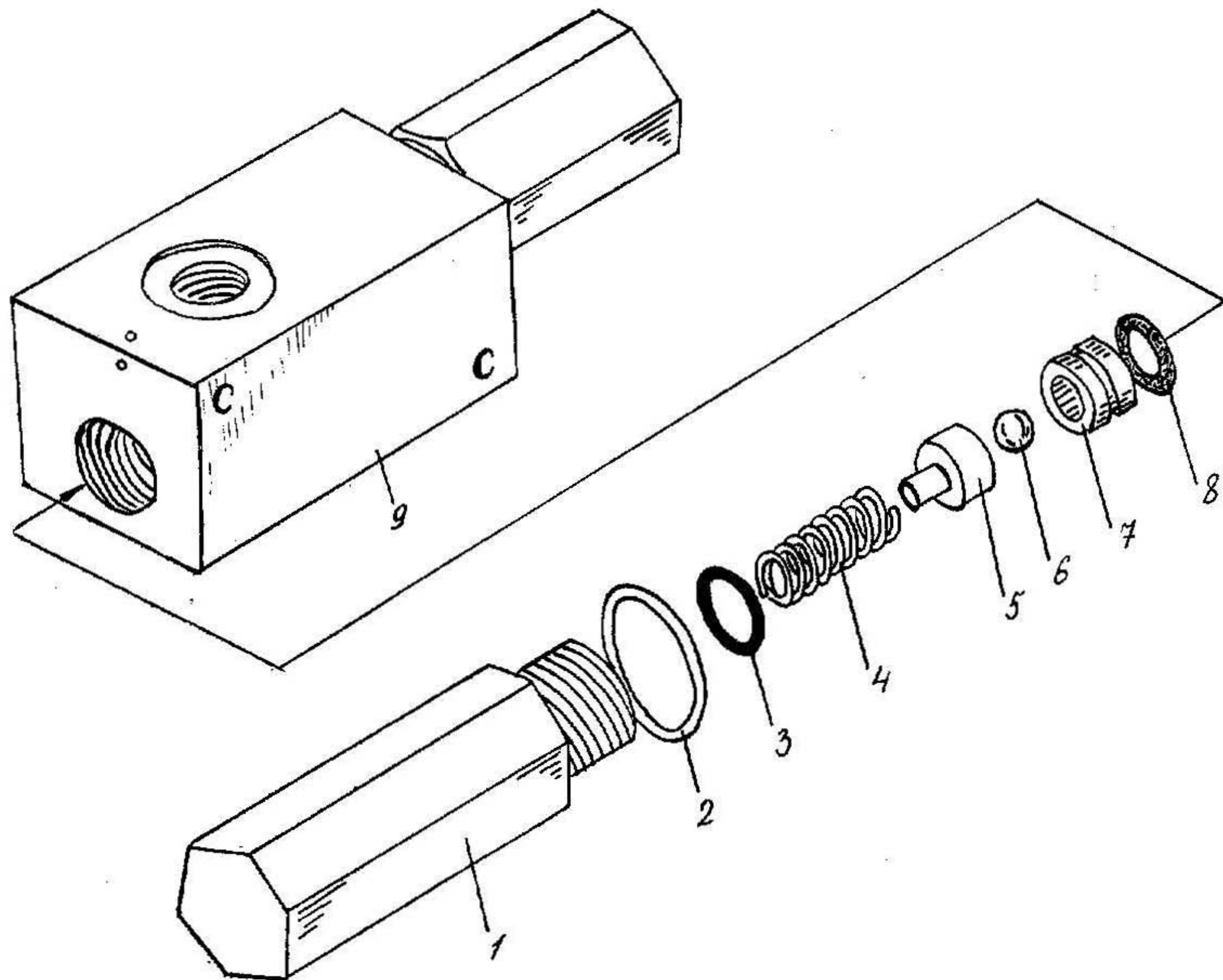
Рис. 30. Гидроклапан перепускной
