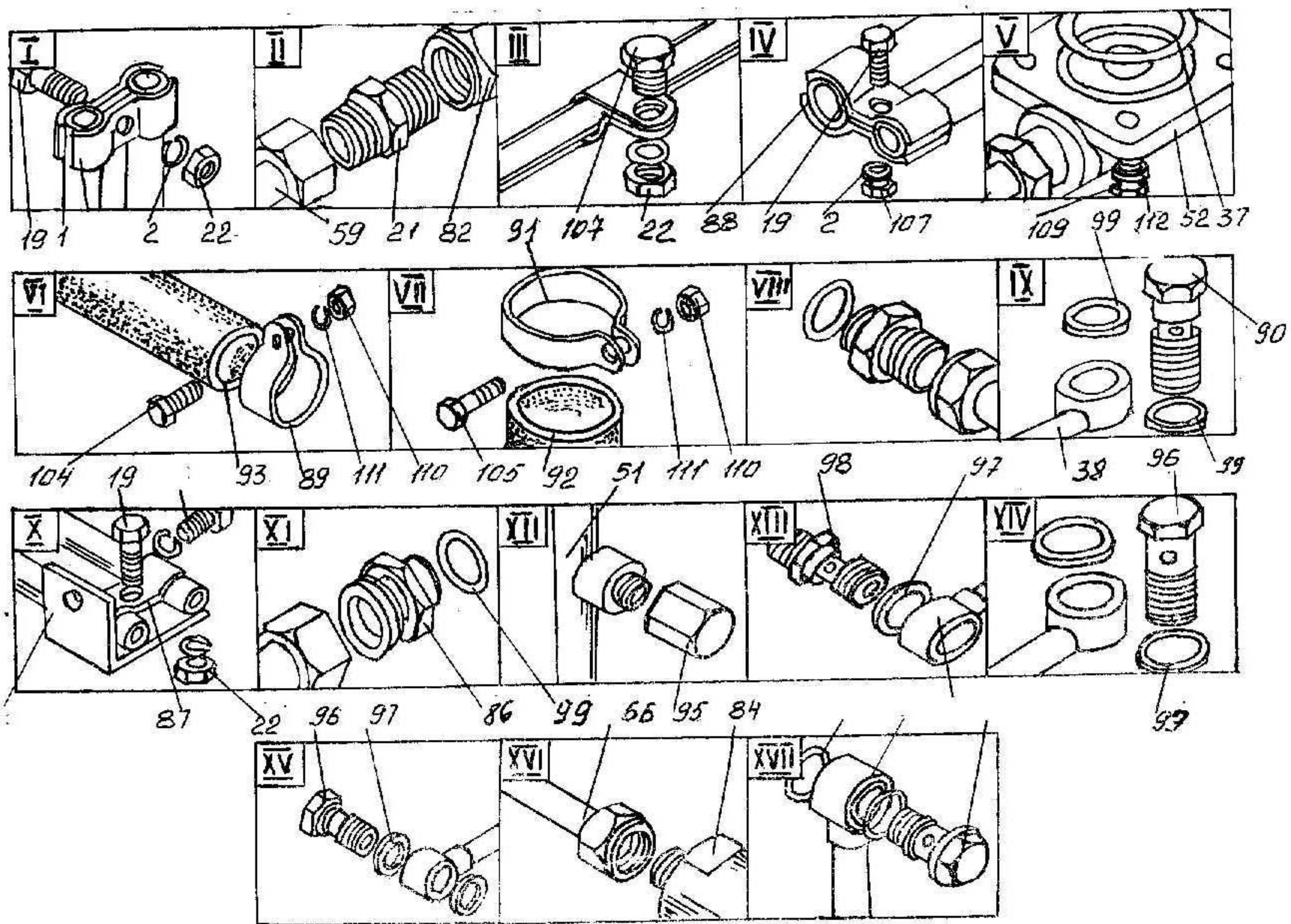
Рис. 28. Гидроразводка
