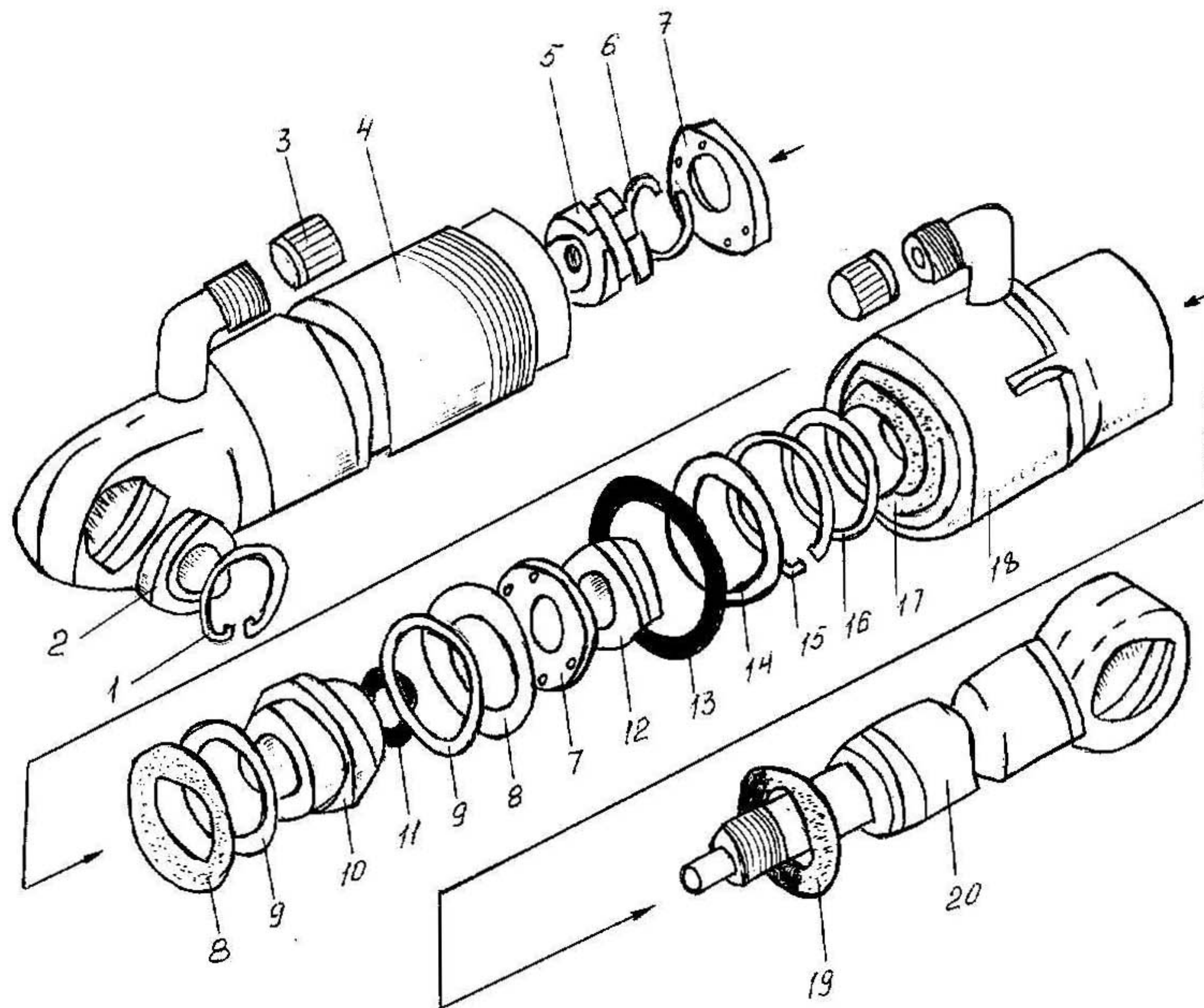
Рис. 8. Гидроцилиндр ковша
