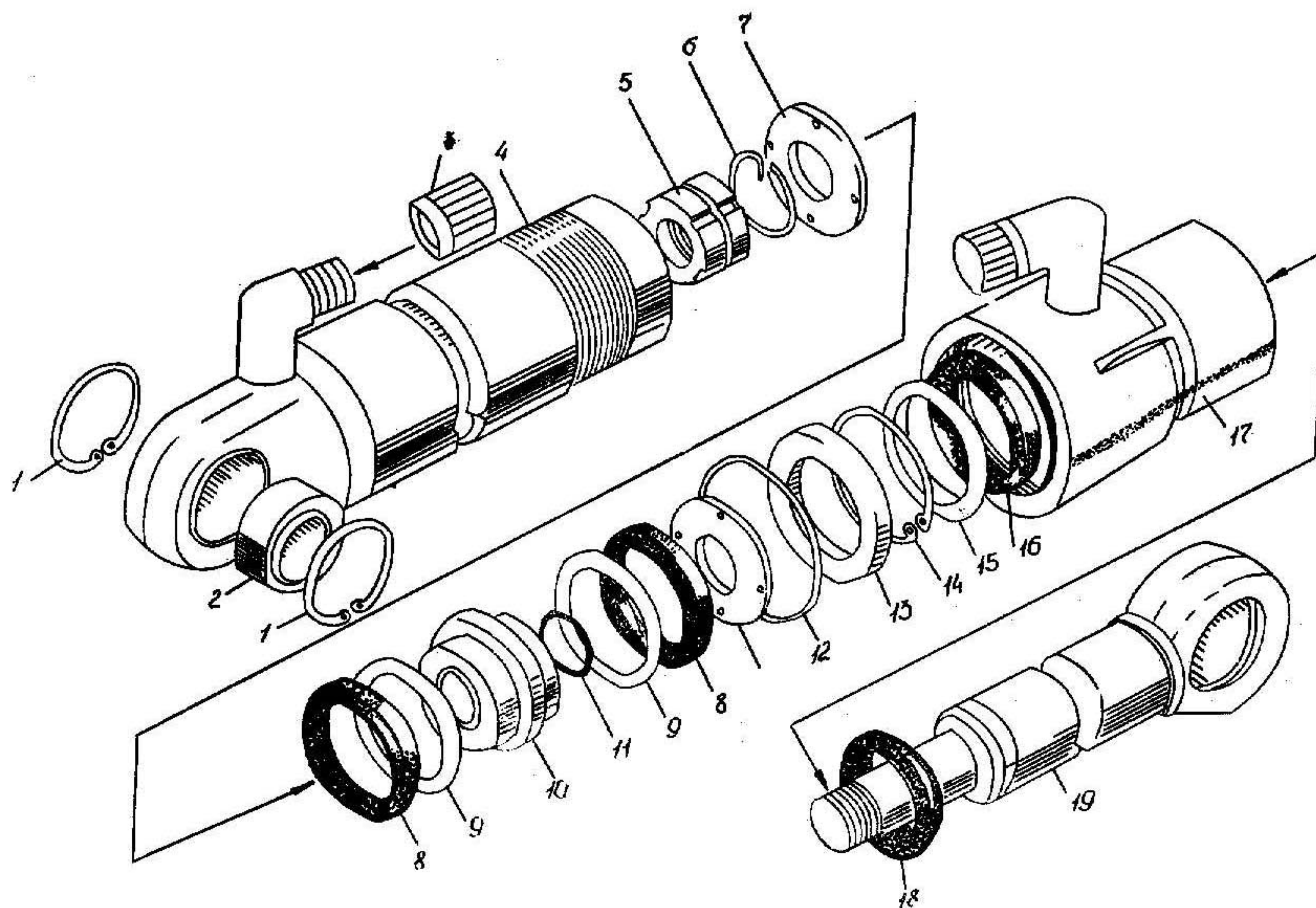
Рис. 19. Гидроцилиндр отвала
