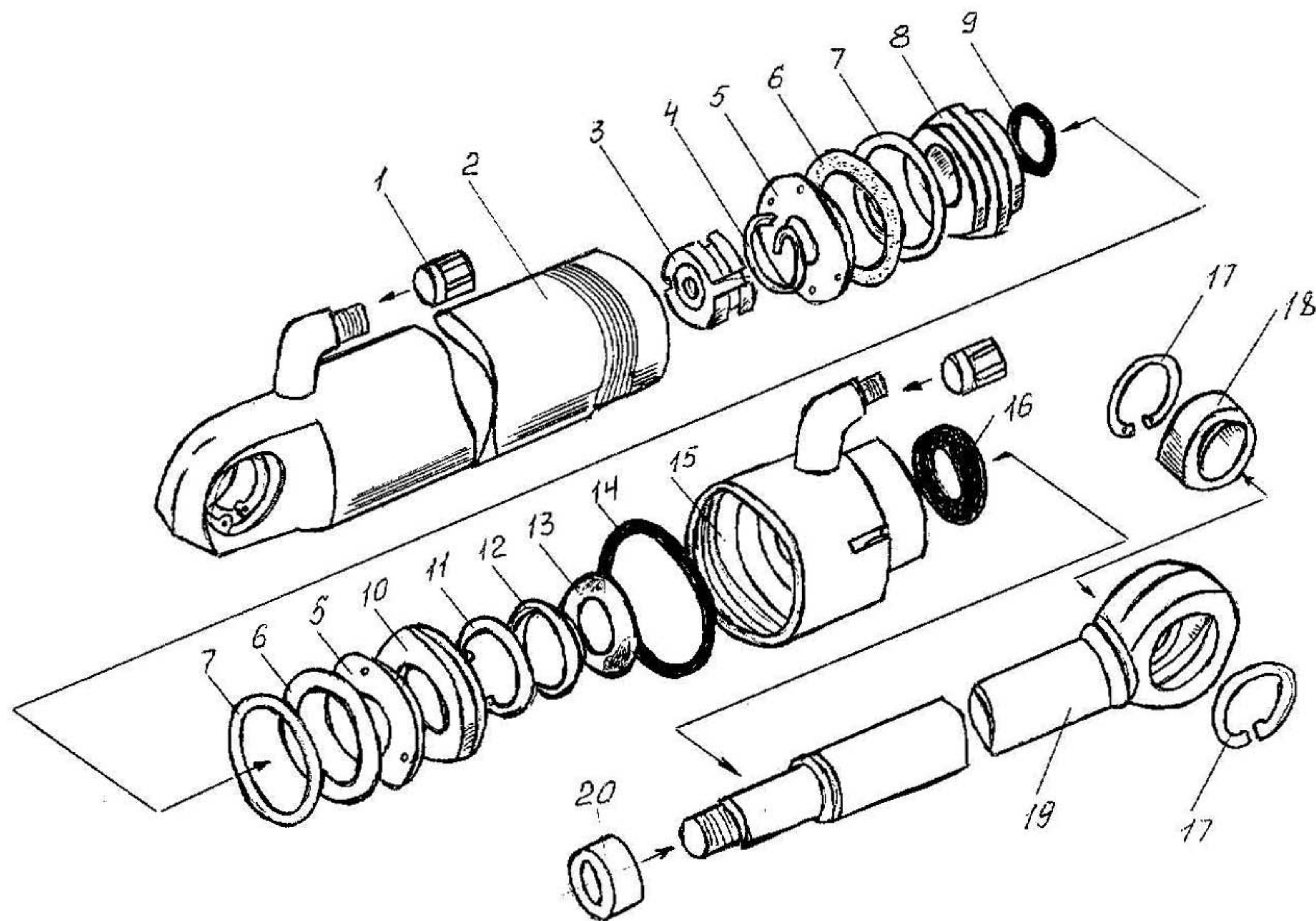
Рис. 18. Гидроцилиндр опорных башмаков
