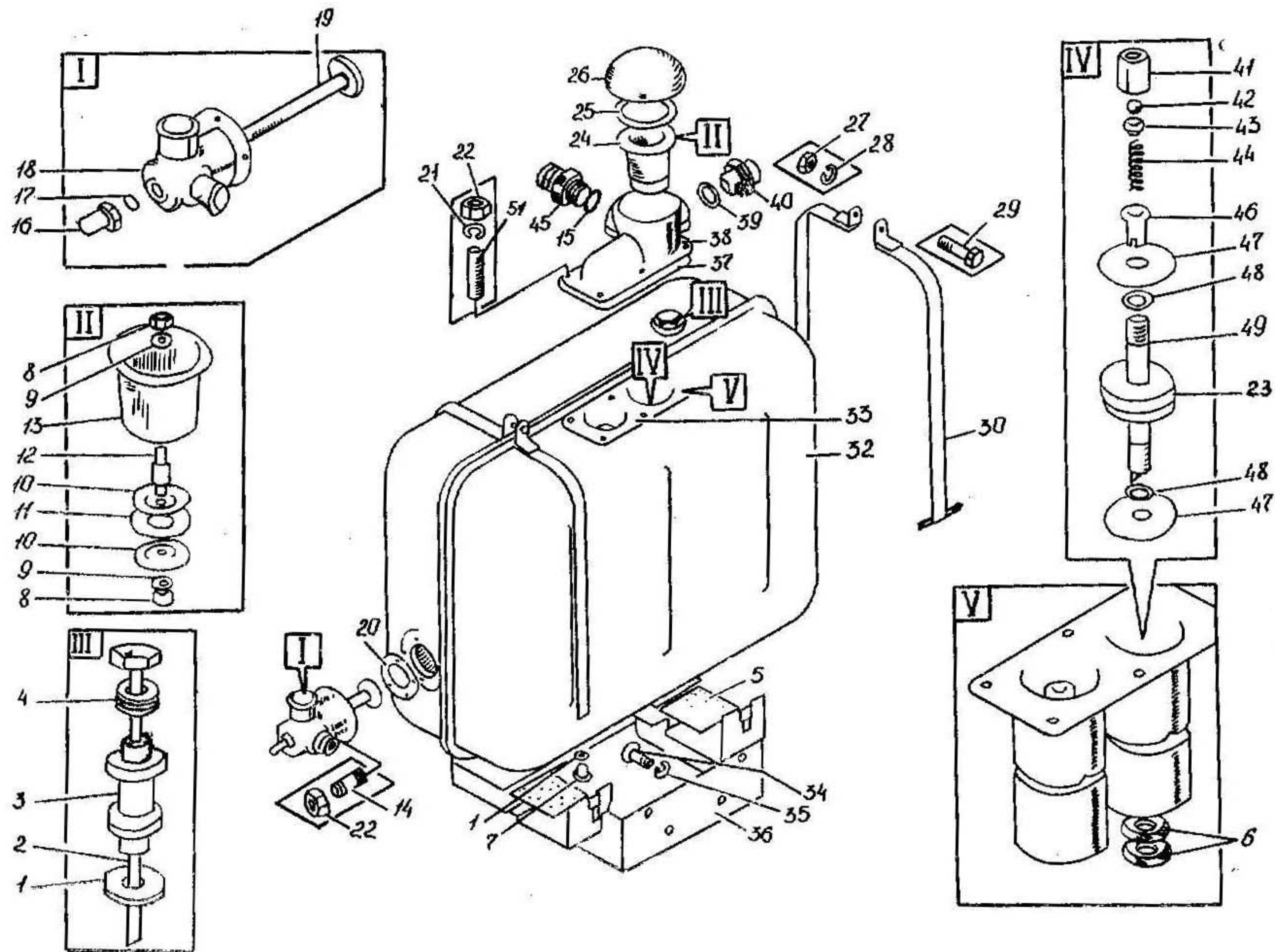
Рис. 14. Бак масляный
