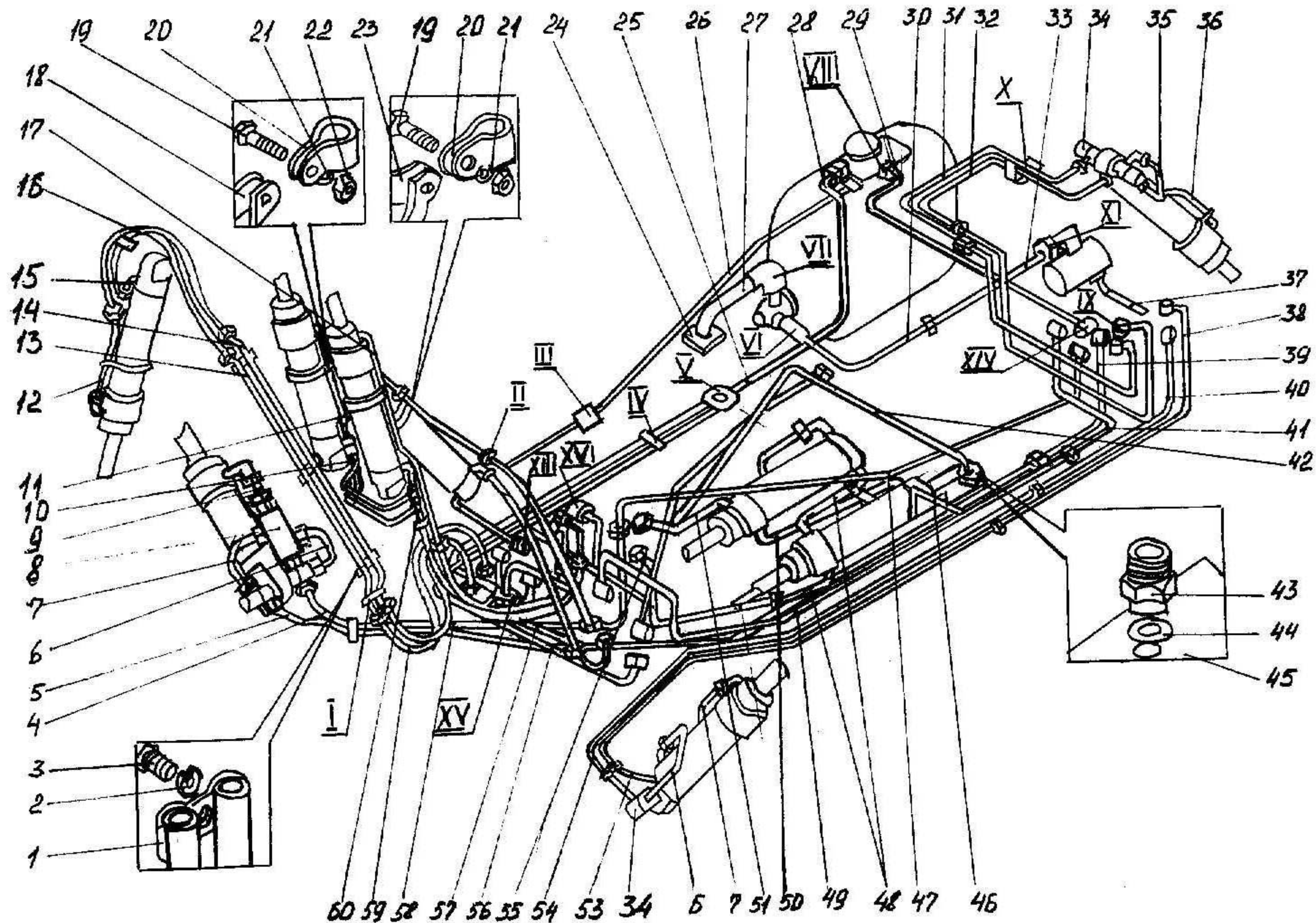
Рис. 26 Гидроразводка
