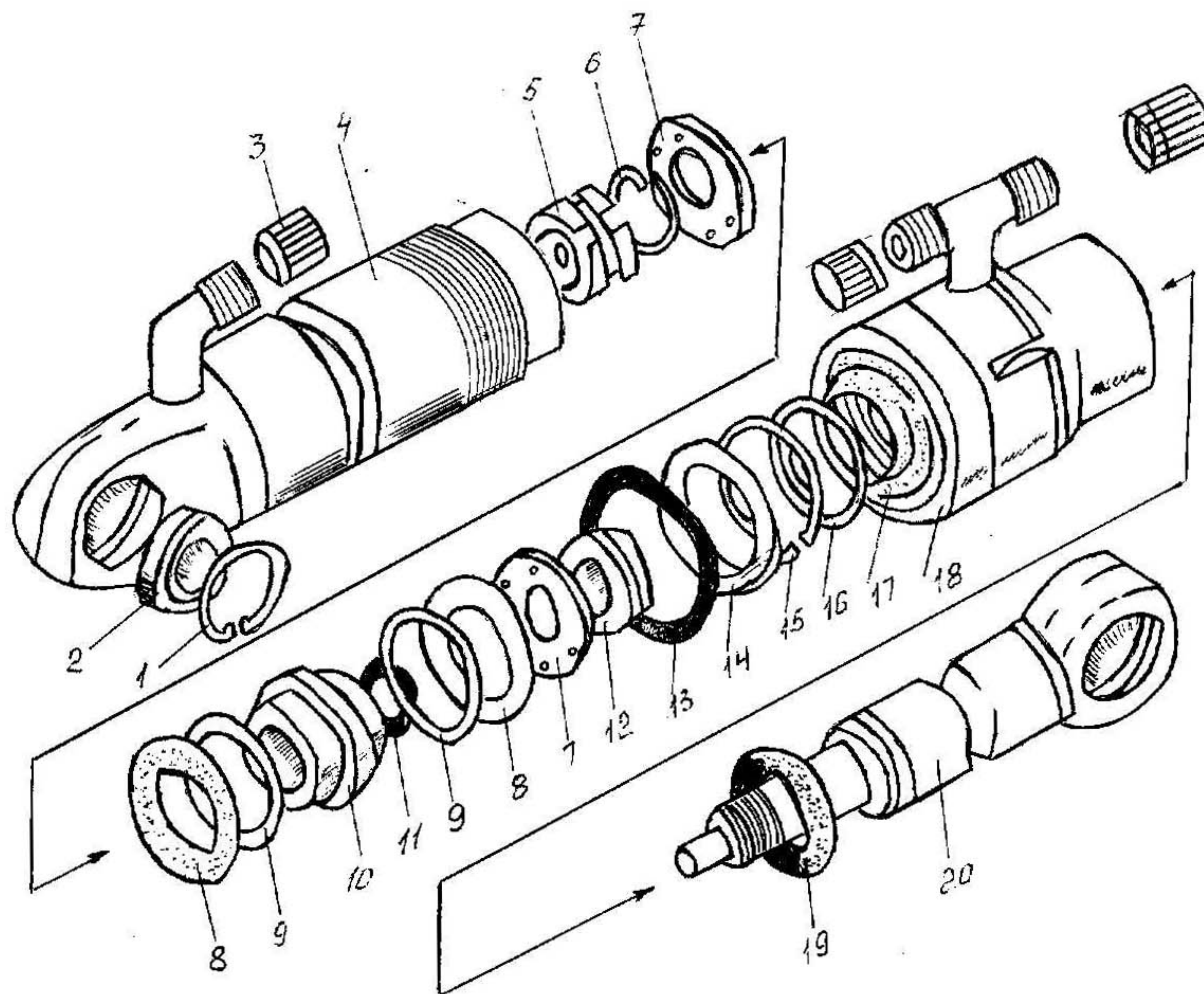
Рис. 10. Гидроцилиндр рукояти левый
